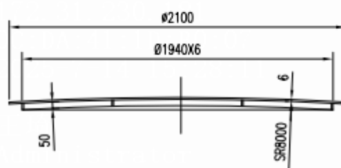
中心顶板详图 不按比例
