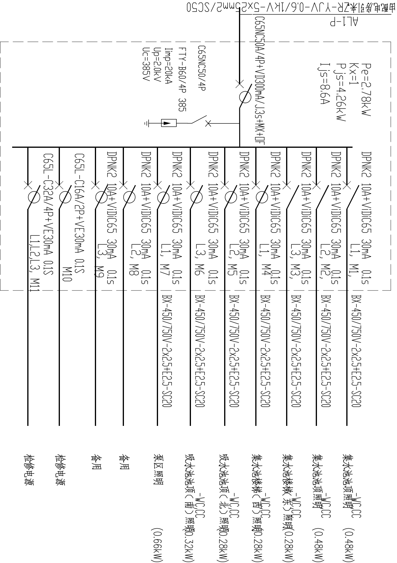
BAL 照明配电箱系统图
