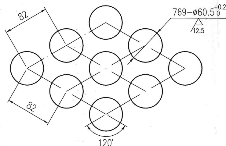
管孔排列详图
