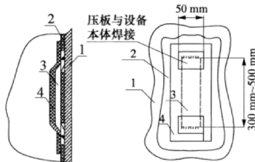
1——设备本体;2——铅衬层;3——钢压板;4——铅盖板
