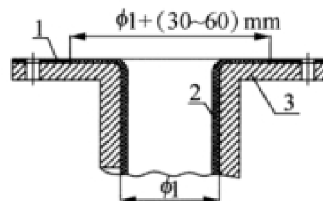
1——已硫化的胶板;2——未硫化胶板;3——设备的法兰
