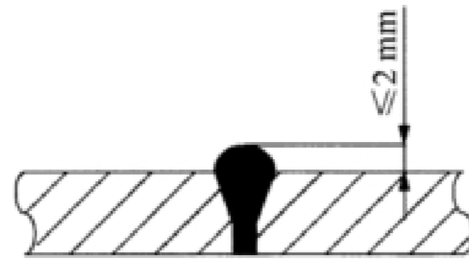
图 3.3.1 对接焊缝
