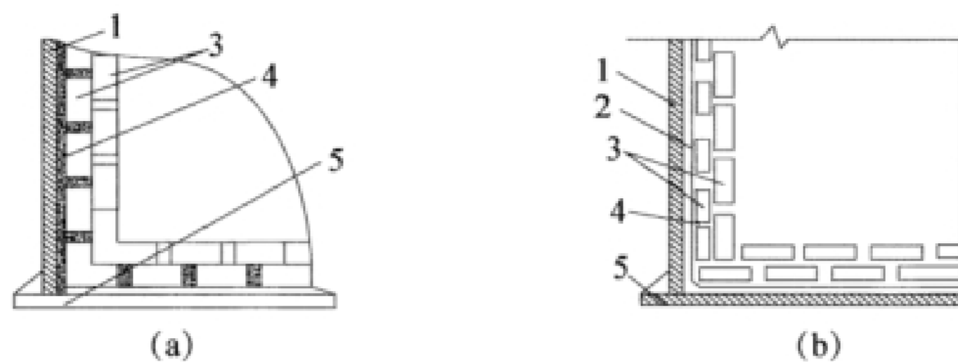
1——设备壳体;2——隔离层;3——砖板;4——胶泥;5——设备底板
