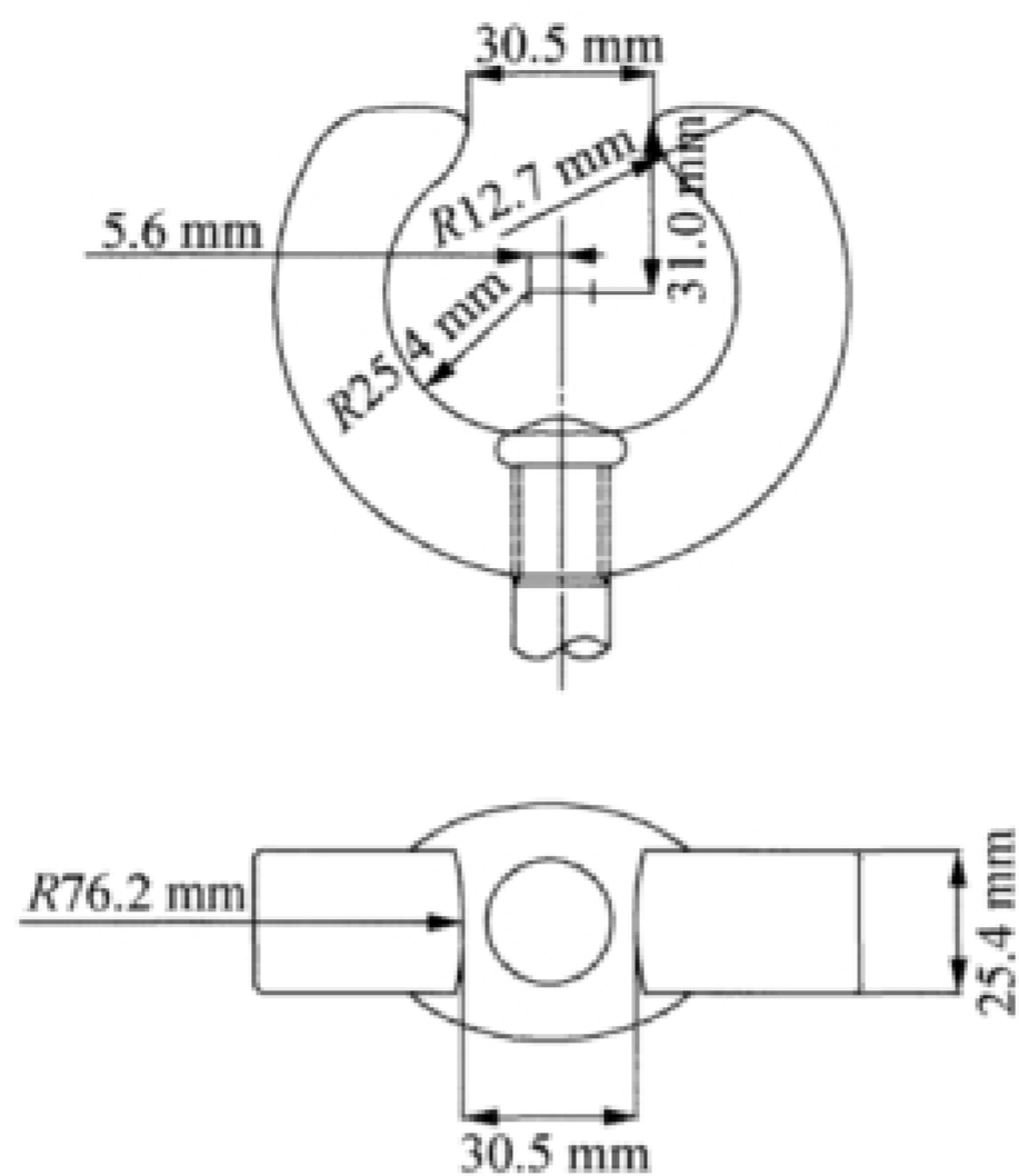
图 B.4.2-2 8 字型试样抗拉强度的夹具
