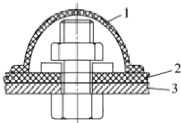
图10 软聚氯乙烯压条螺钉固定法衬里
