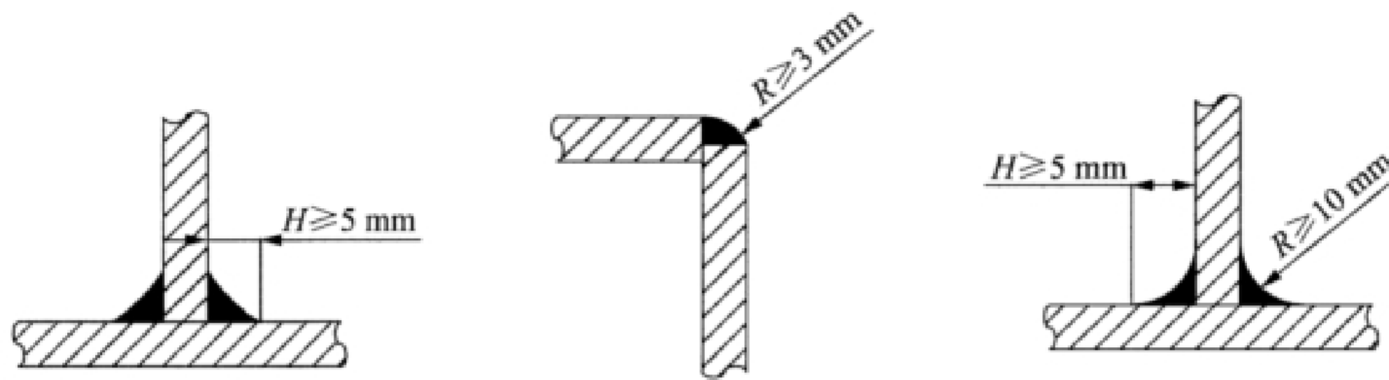
图 3.3.3-1 角焊缝 图 3.3.3-2 凸出角焊缝 图 3.3.3-3 内角焊缝
