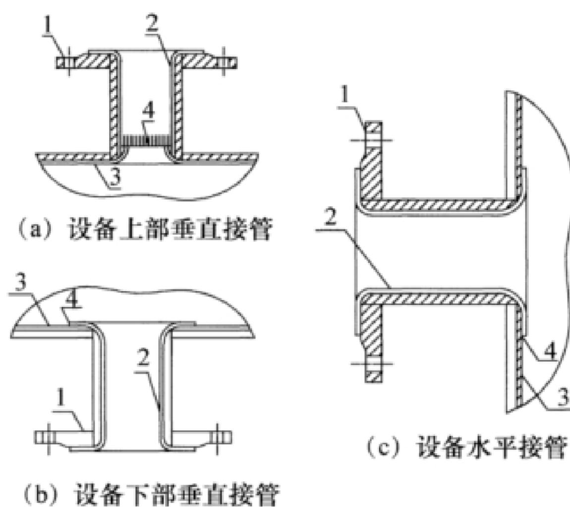
1——设备孔；2——孔衬铅板；3——衬铅板；4——焊缝
