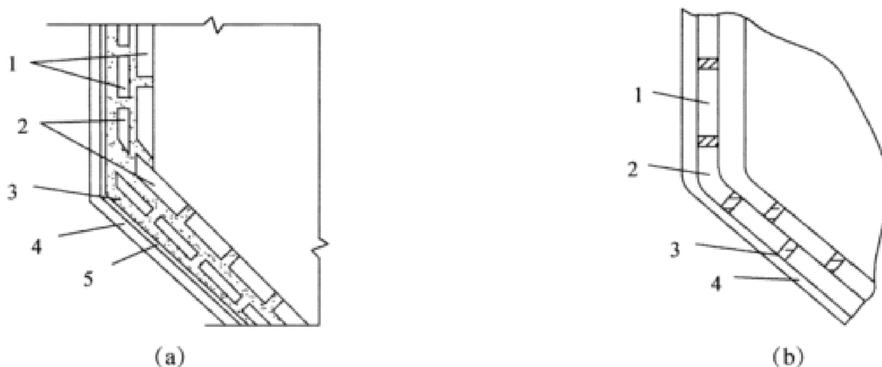
图 2 设备椭圆形封头与筒体衬砖板连接方式
