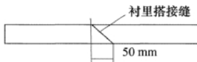
图 12 搭接结构
