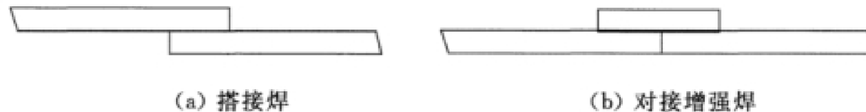
图 8.4.4 板-板焊接型式
