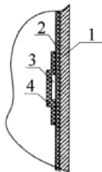
1——设备本体;2——衬铅板;3——钢压条;4——铅防护条
