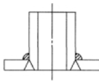
图 8.4.3-2 圆筒与支管焊接型式
