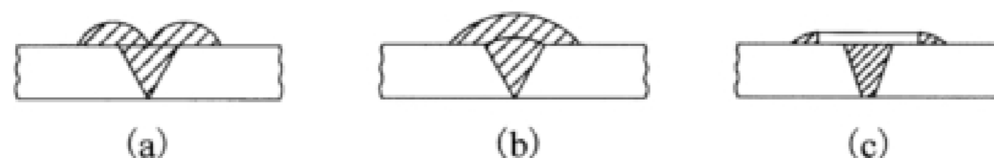
图 8.4.3-1 板-板焊接形式
