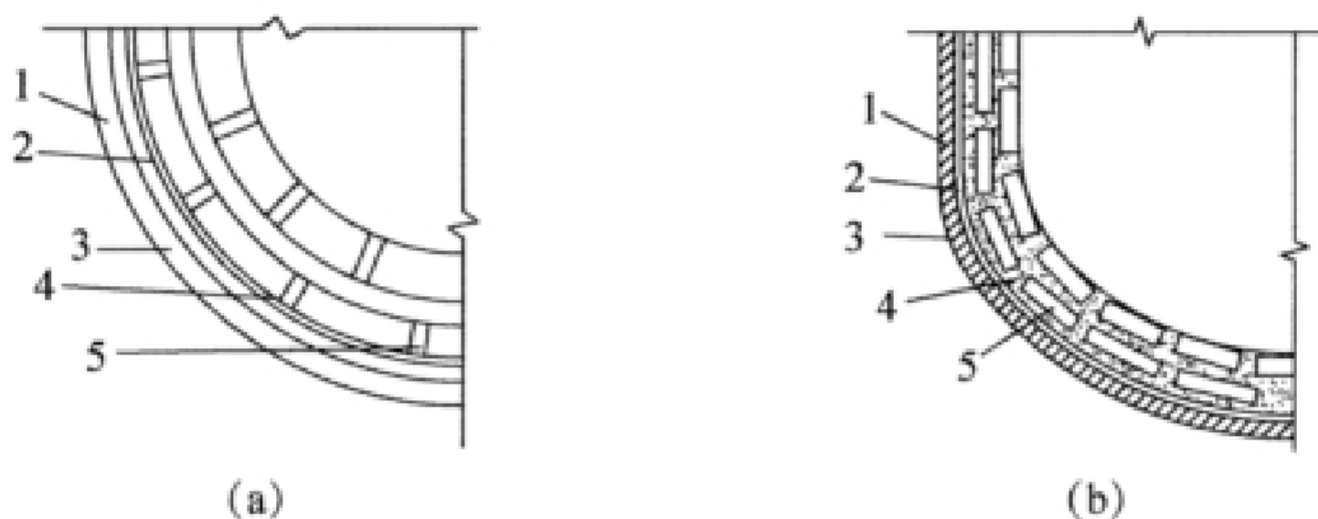
图 1 设备平底与筒体衬砖板连接方式
