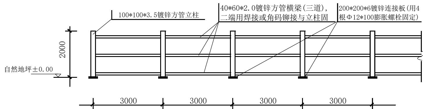
围挡构造示意图
