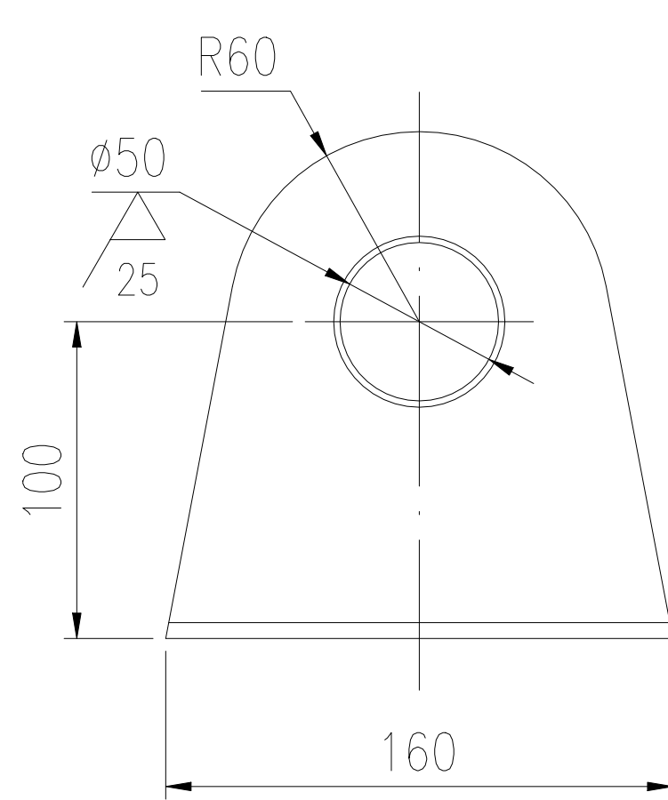
件1详图 1:4
