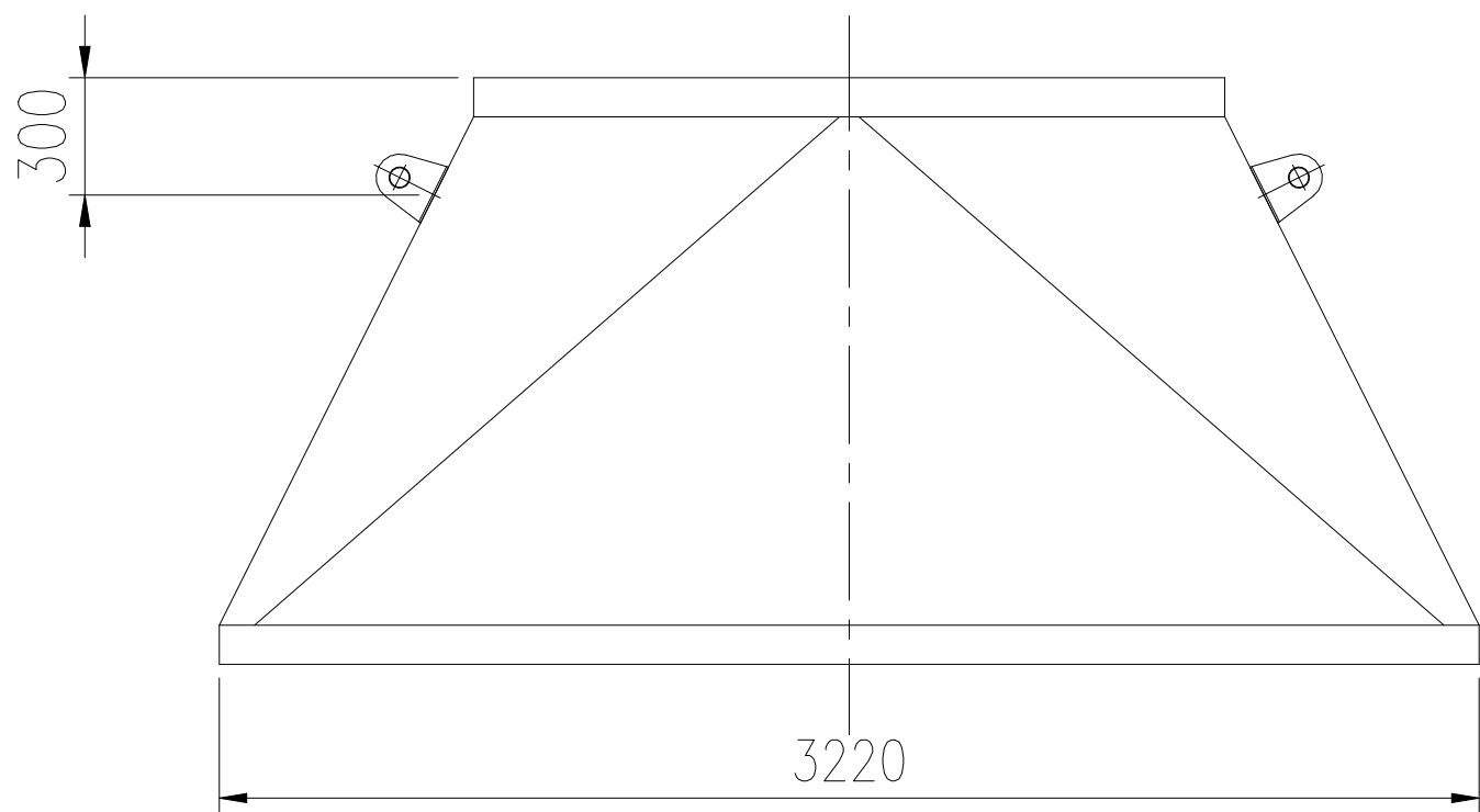
件1详图 1:4
