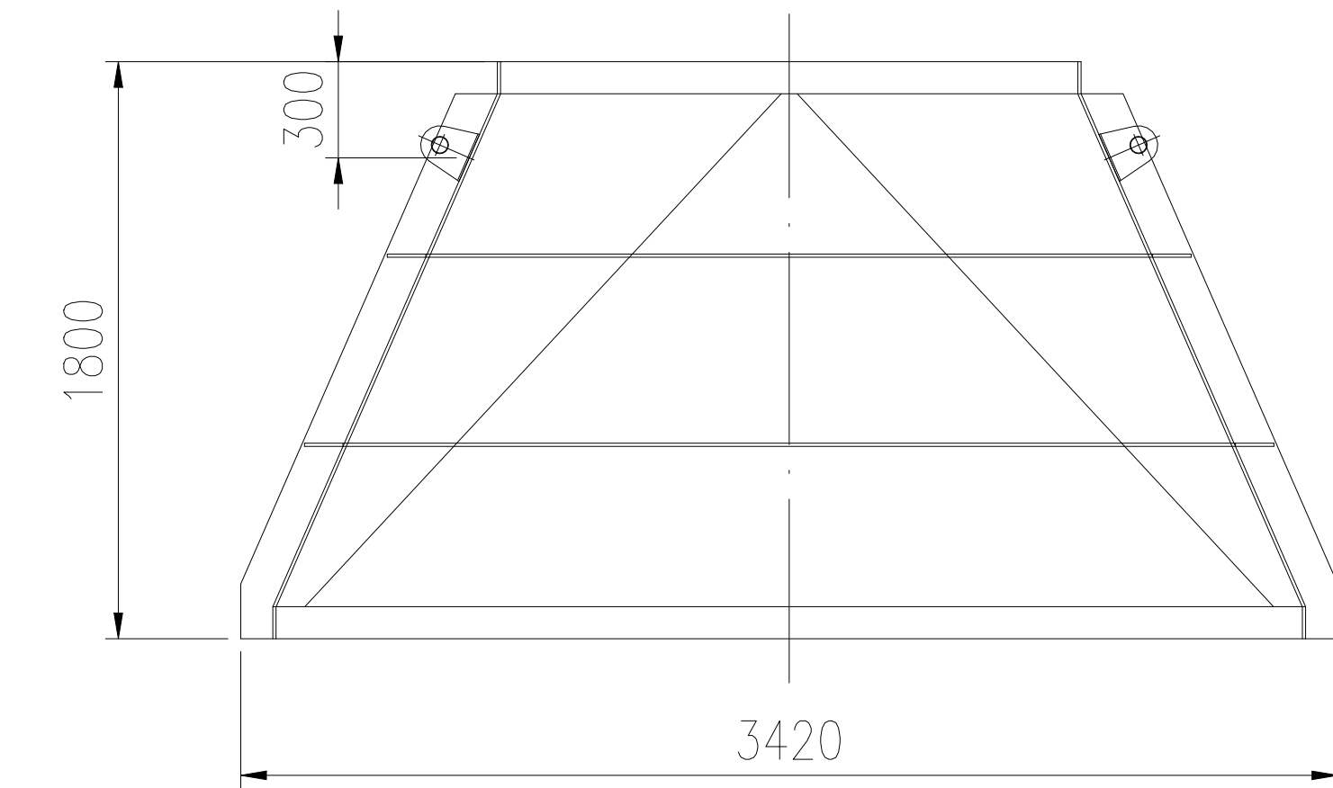
件1详图 1:4
