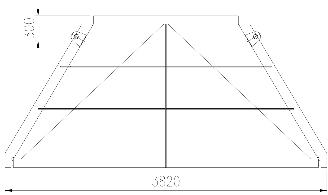
件1详图 1:4
