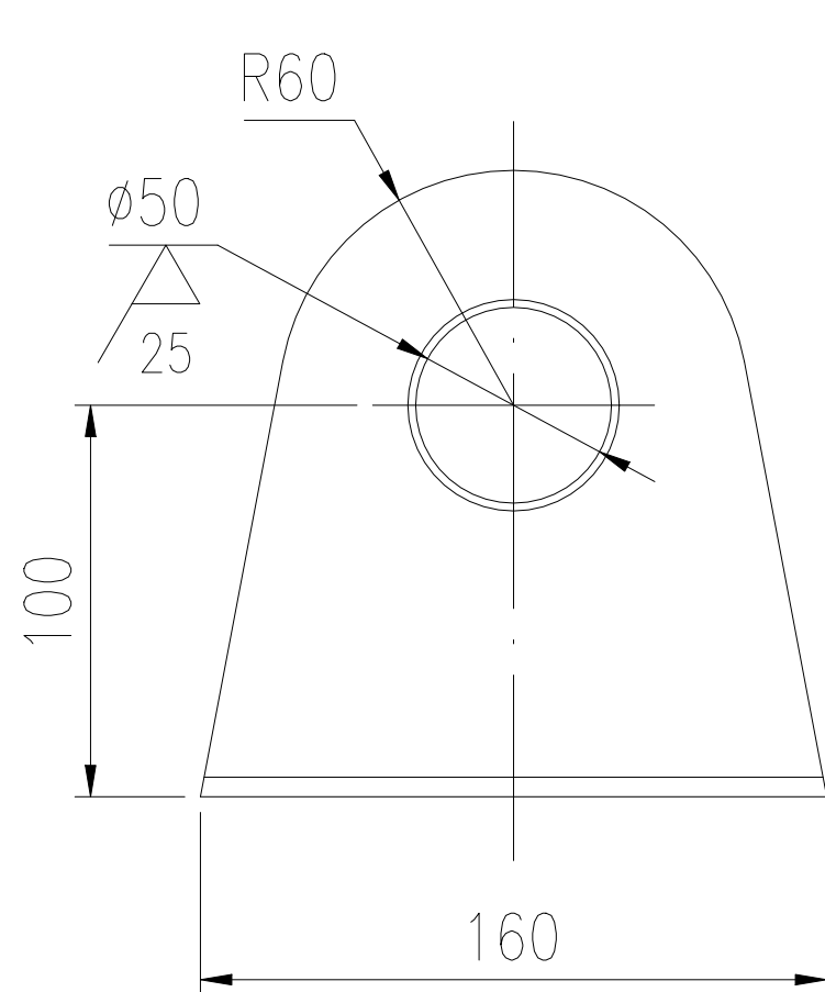
件1详图 1:4
