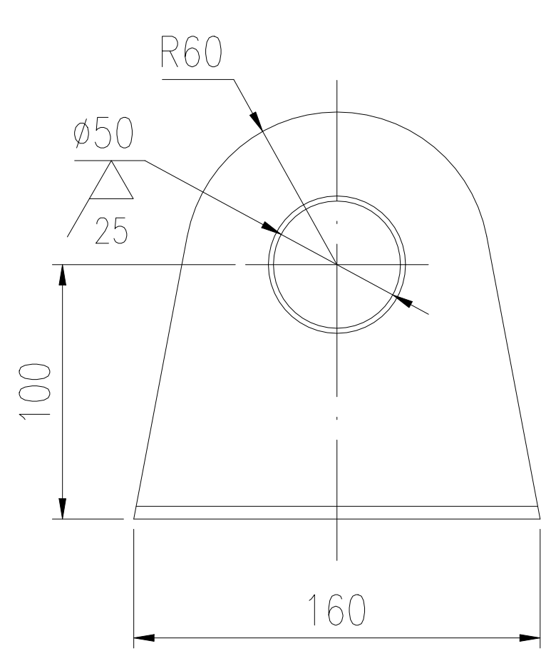
件1详图 1:4
