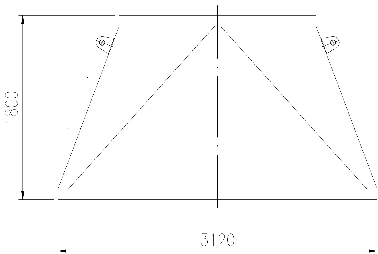
件1详图 1:4
